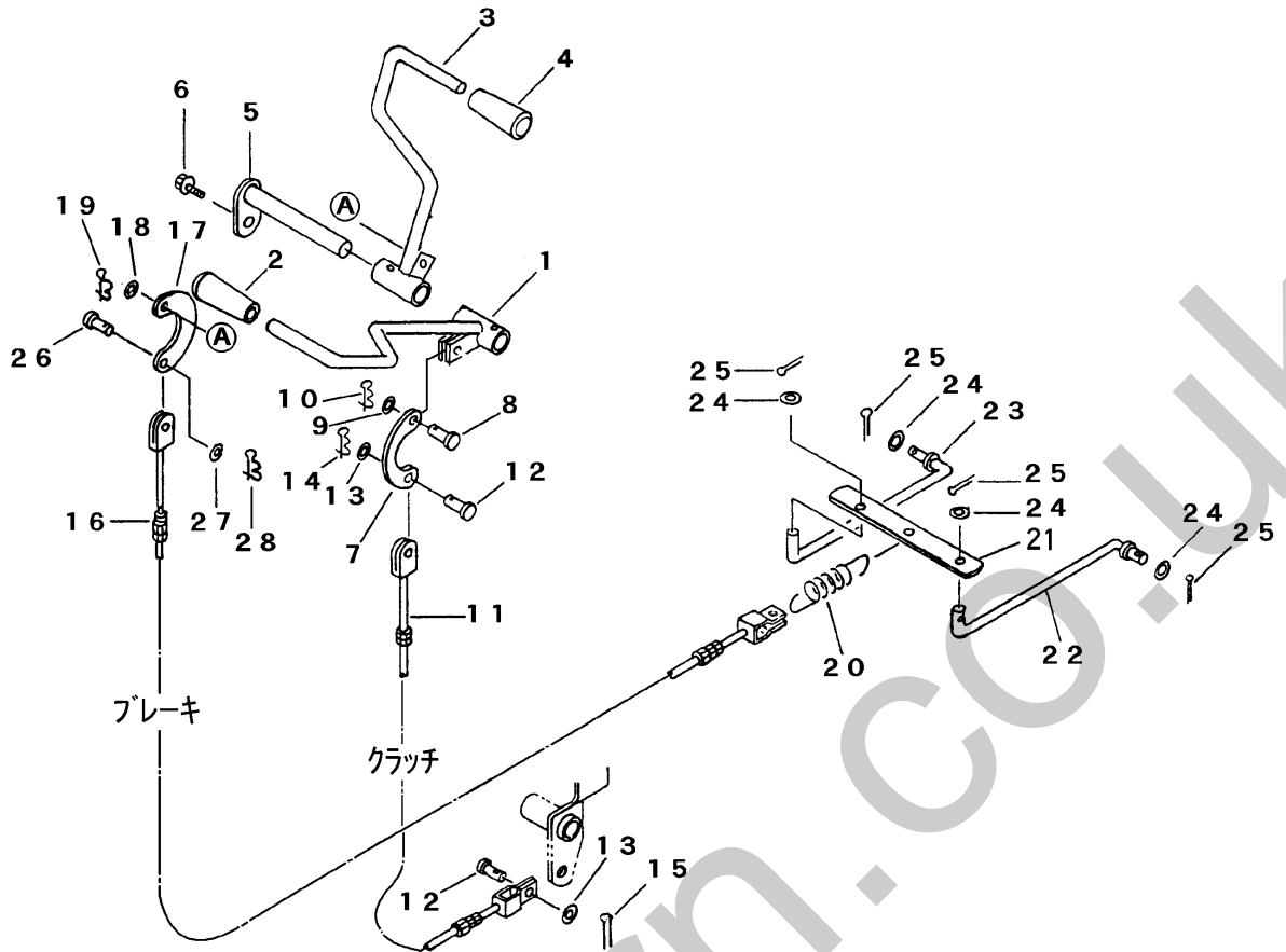
FIG 15 クラッチ・ブレーキ CLUTCH・BRAKE
