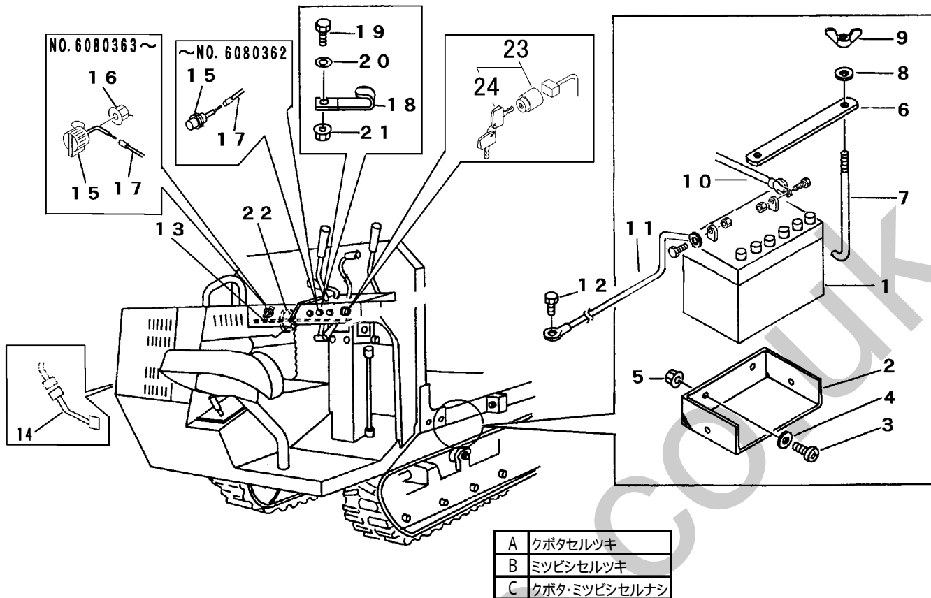
FIG 5 デンソウ (箱型・ダンブ) ELECTRIC EQUIPMENT
