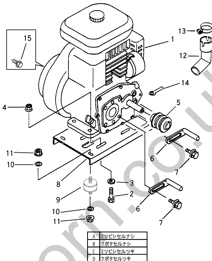
FIG 1 エンジン（短尺材用荷台・箱型） ENGINE
