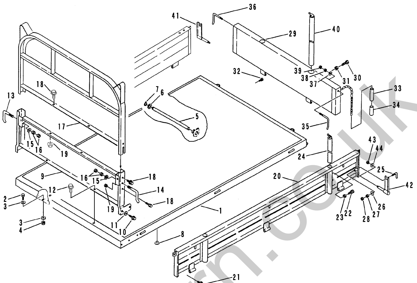
FIG 22 ニダイ & ゲート (箱型三方開ショート) WAGON & GATE
